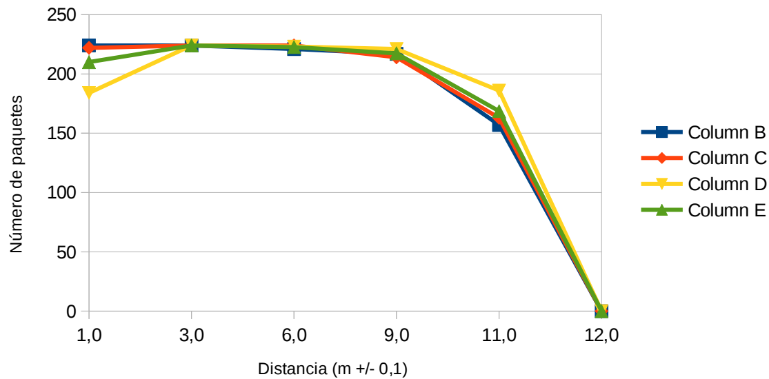
1/4 Onda sin plano de tierra - 5V
