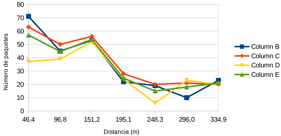
1/4 Onda plano de tierra 5° - 12V
