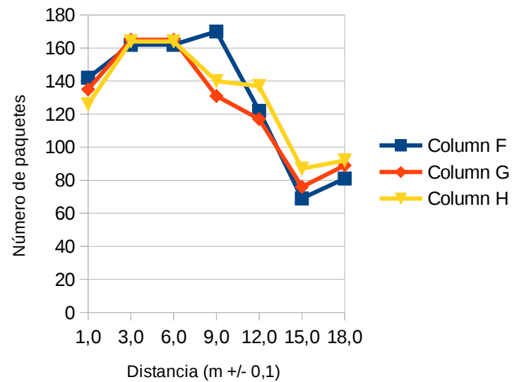
1/4 Onda con plano de tierra a 0°
