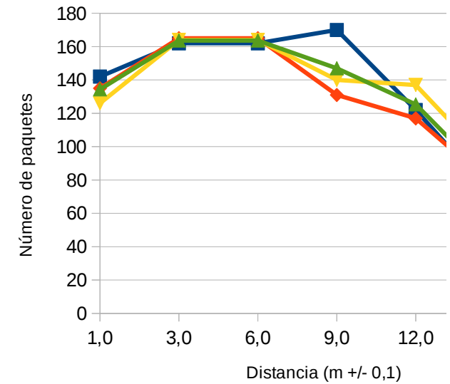
1/4 Onda con plano de tierra
