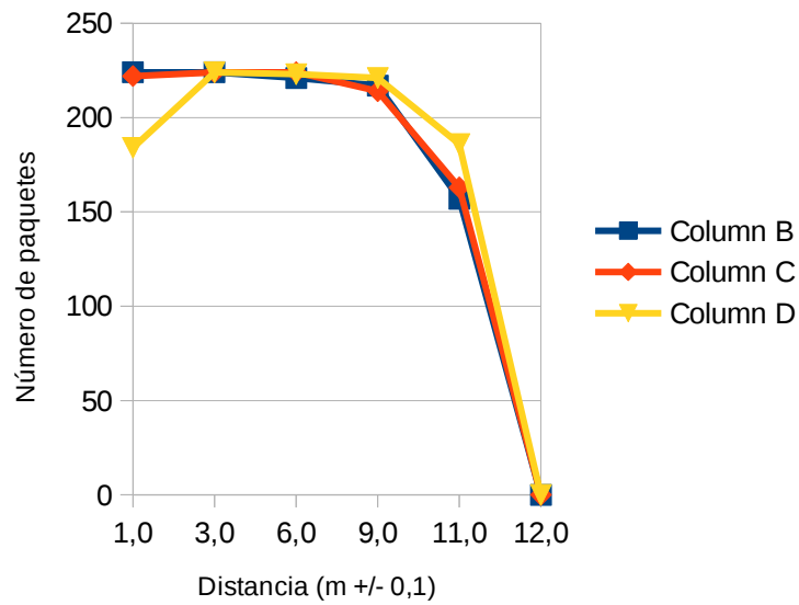
1/4 Onda sin plano de tierra
